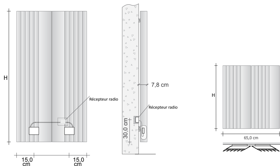
Version mixte
