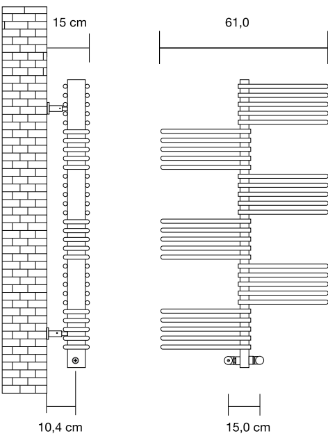
Entraxe raccordements avec mesures en référence aux vannes Tubes
