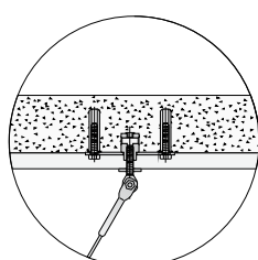
Détail « B » Pour structure en BRIQUES
