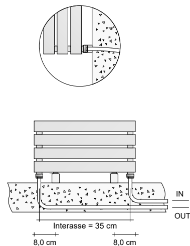
Schéma RACCORDEMENTS MV#170 et MV#140
