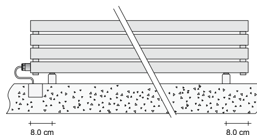
Branchement ÉLECTRIQUE mod. MOEC#080
